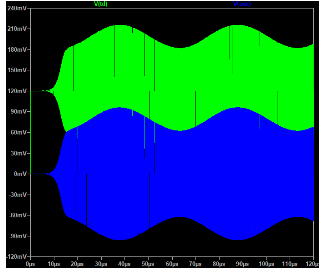
图 15 LTspice 仿真结果
