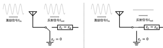
图 1 背散射通信机理
