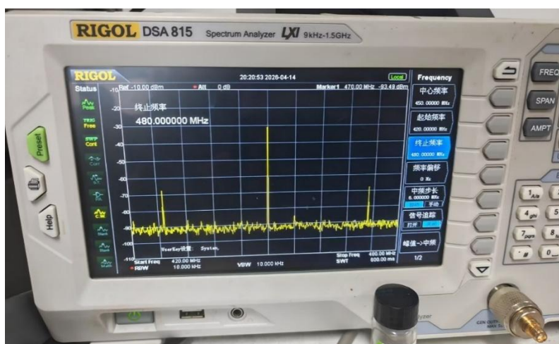
图 4 散射后频谱图
