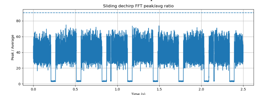
图 5 FFT 峰值检测结果(风扇转动)
