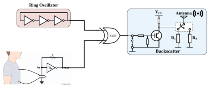
图 8 标签端设计图
